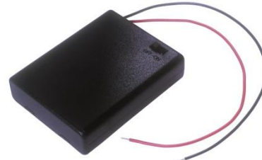
SBH441AS (スイッチ、カバー付き)
